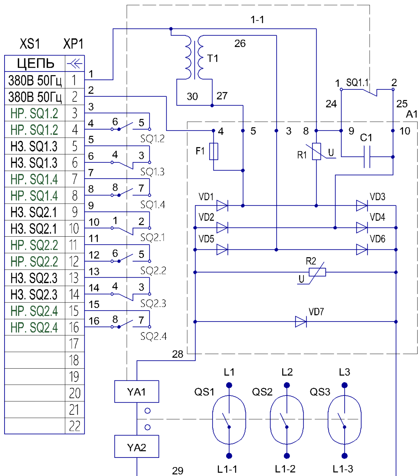
Рисунок 2 - Схема электрическая принципиальная контактора КВТ-1,14-2,5/250 на номинальное напряжение цепи управления 380 В переменного тока
