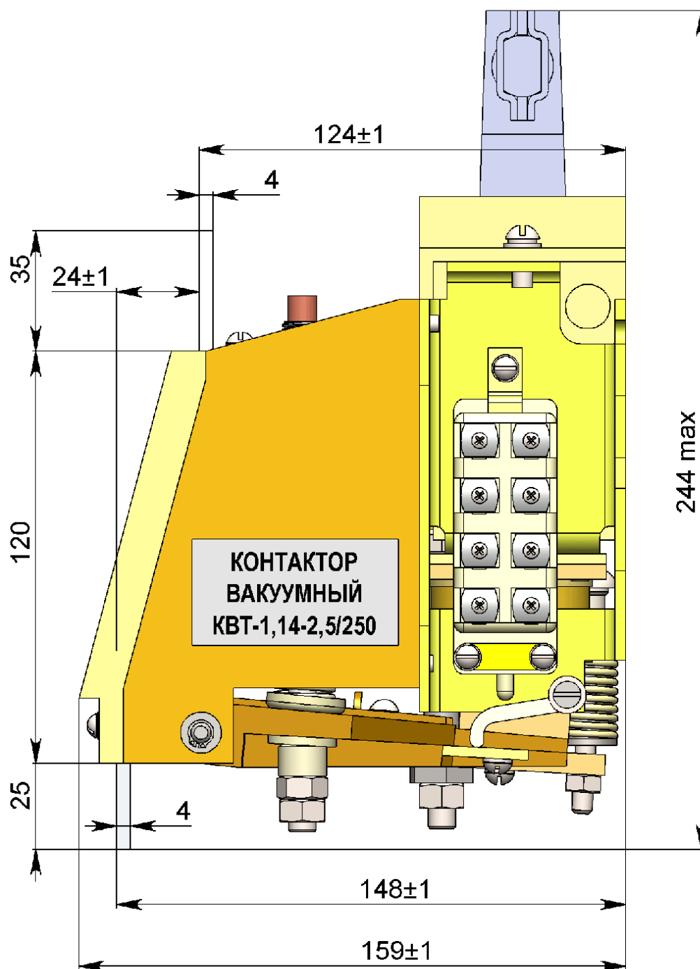
Чертеж 1 КВТ-1,14-2,5/250 Вид справа габаритные, справочные и присоединительные размеры
