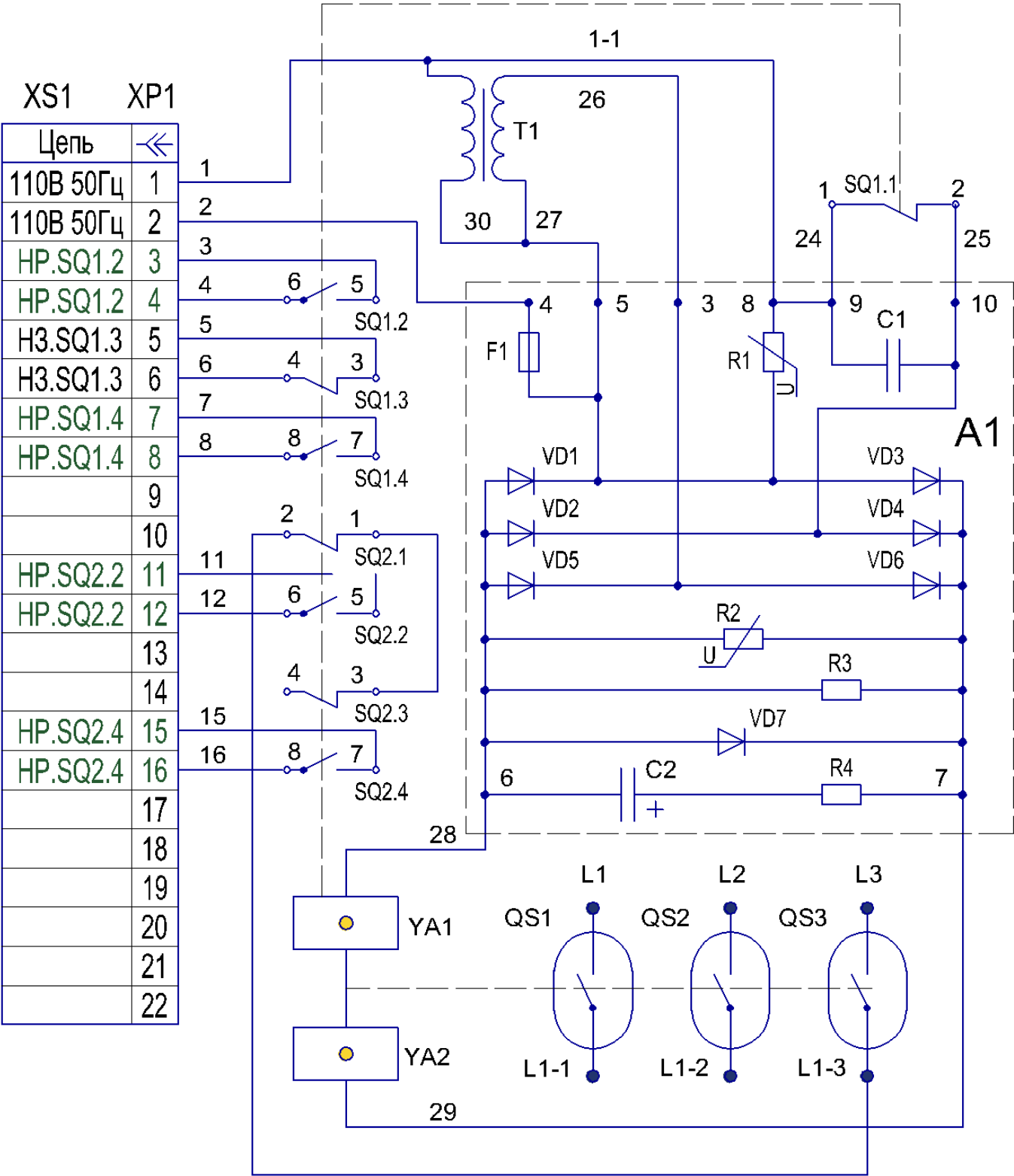
Рисунок 5 Принципиальная электрическая схема вакуумного контактора КВТ-1,14-2,5/250 в исполнении из трекингстойкой пластмассы
