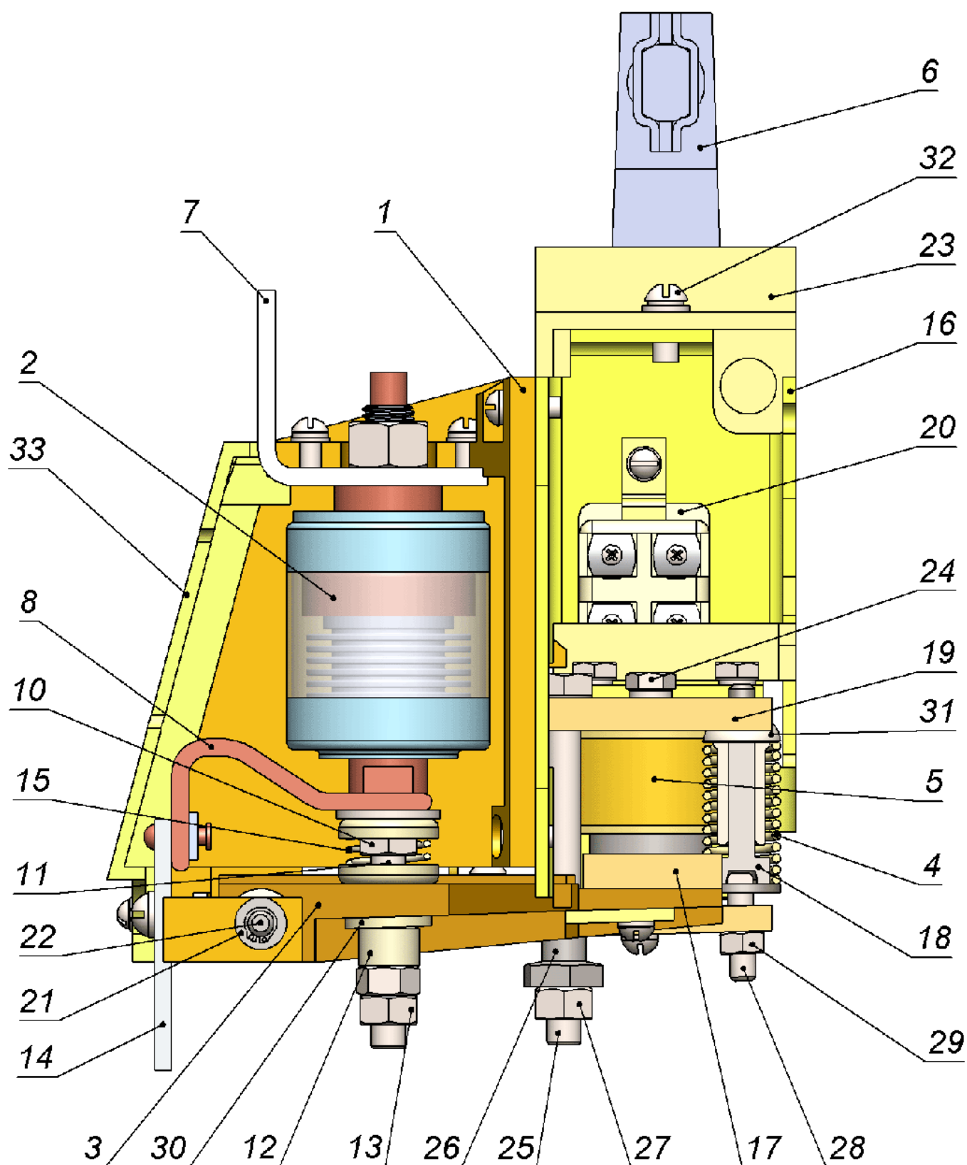
Чертеж в разрезе Устройство и работа контактора КВТ 250
